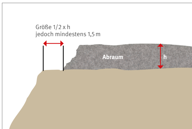
Abb. 3 Schutzstreifen bei Abraubeseitigung von Hand
