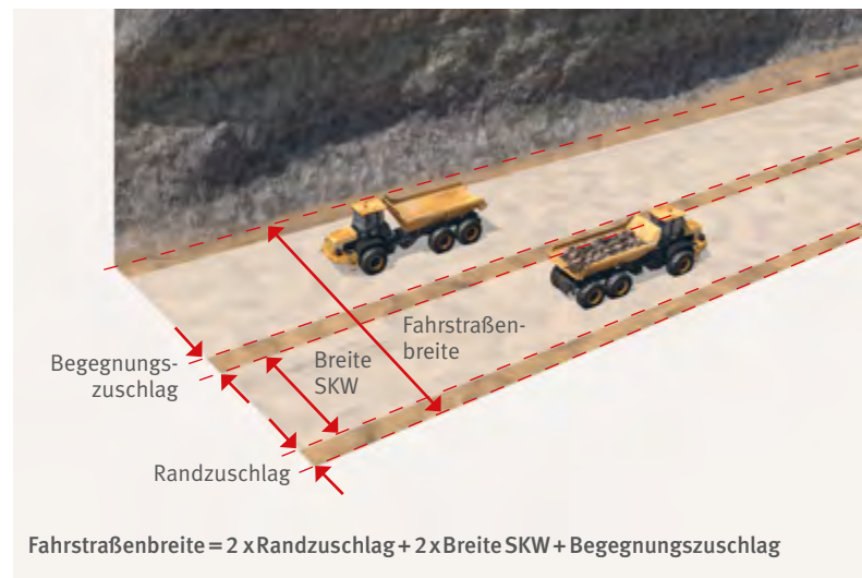
Abb. 4 Berechnung Mindestbreite der Fahrstraßen
