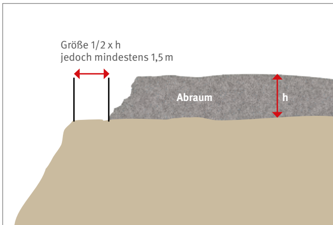
Abb. 2 Schutzstreifen bei Abraumbeseitigung von Hand
